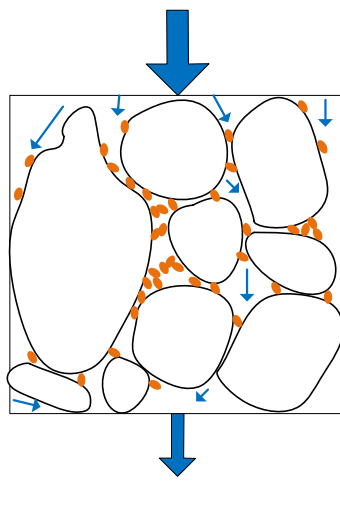
固化能力を持つ微生物の栄養、固化成分を浸透させ、砂の間隙中に結晶鉱物を析出させ強度増進(出砂抑制)効果を得る。
