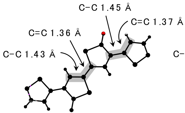
PBTDT4 のモデル化合物
