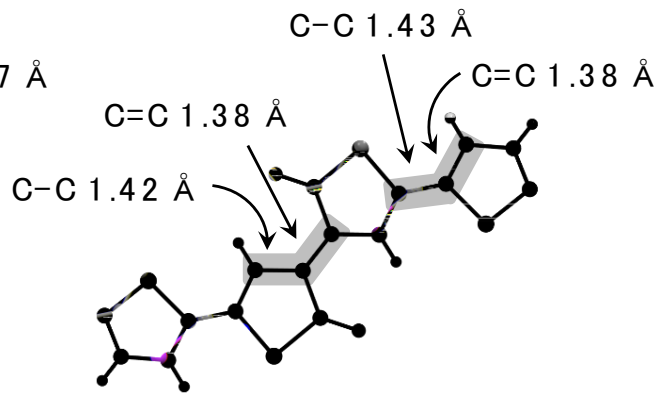
PSP4T のモデル化合物
